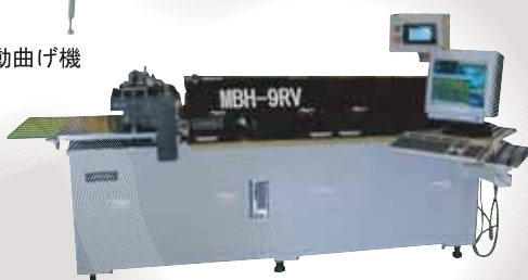
超振動拔型刃物自動曲げ機 真空成型向け
